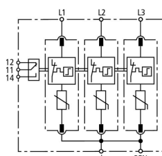
Prinzipialschaltbild VT2 M TNC 320 FM AT
