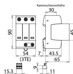
Maßbild VT2 M TNC 320 FM AT
