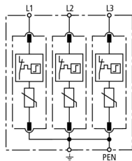
Prinzipschaltbild VT2 M TNC 320 AT
