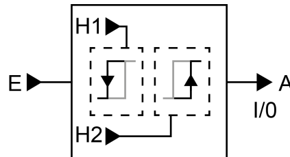
Bild 31: Grenzwertschalter
