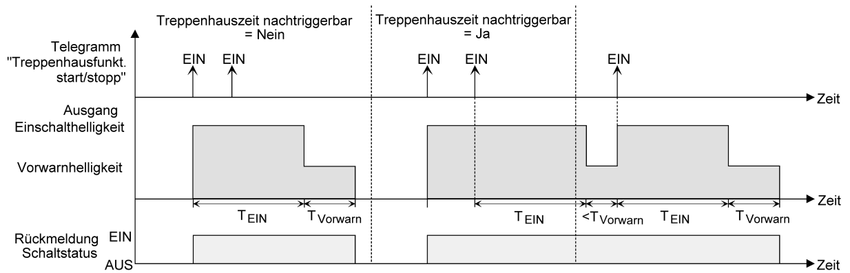
Bild 16: Einschaltverhalten der Treppenhausfunktion ohne Soft-Funktionen
