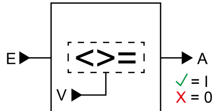
Bild 29: Vergleicher
