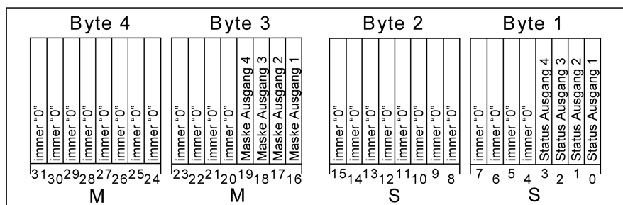
Bild 13: Struktur des Objekts "23" der Sammelrückmeldung für die Ausgänge 1 ... 4
