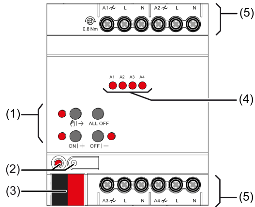
Bild 1: Geräteaufbau
