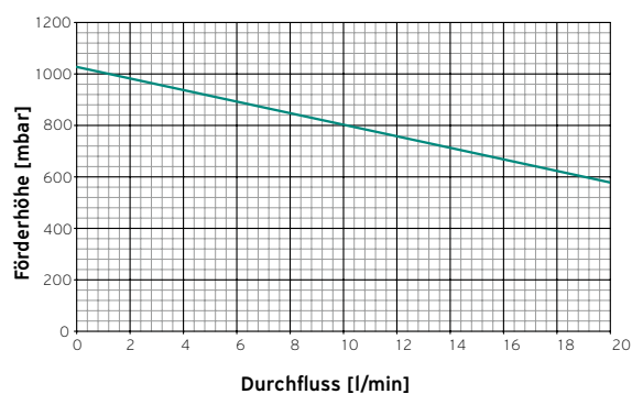
Kennlinie VMS 70
