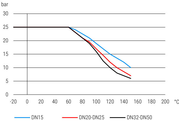
Druck-Temperatur-Diagramm
