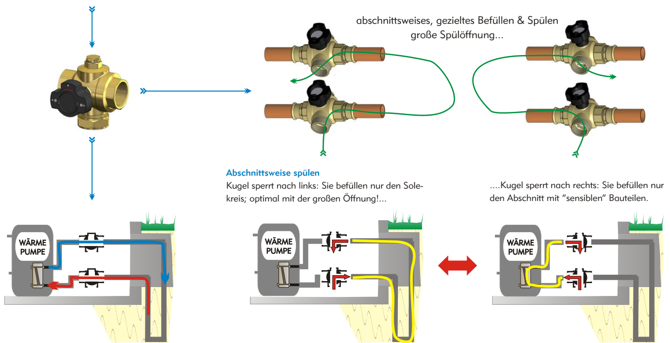
4-Wege-Kugelhahn mit T-Bohrung...
