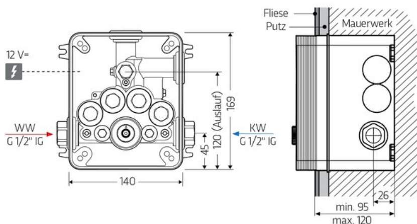
Montage: Maße in cm
