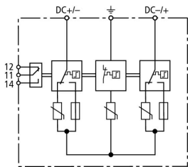
Prinzipschaltbild DG YPV SCI 1000 FM
