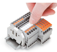
Einrasten eines WMB-Beschriftungsstreifens in die Beschriftungsaufnahme
